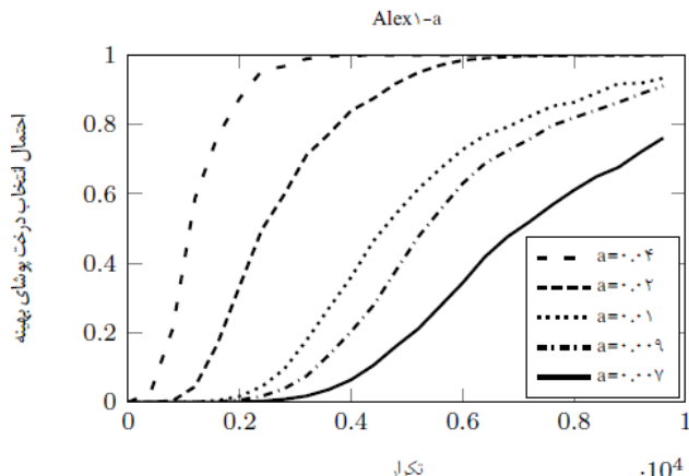
شکل ۸: نحوه تغییر احتمال انتخاب درخت پوشای کمینه در الگوریتم ۱ به ازای مقادیر مختلف نرخ یادگیری.
