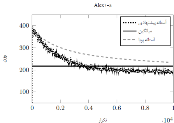
شکل ۳: مقایسه مقادیر مورد استفاده در ارزیابی اقدامات یادگیری آتاماتا در الگوریتم ارائه شده در [۱۶] و الگوریتم ۱ پیشنهادی در مقایسه با میانگین وزن درخت پوشای بهینه (نرخ یادگیری ۰/۰۰۷ بوده است).
