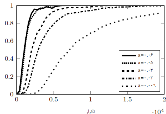
شکل ۱۰: نحوه تغییر احتمال انتخاب درخت پوشای کمینه در الگوریتم ۱ به ازای مقادیر مختلف نرخ یادگیری. (در متن ارجاع ندارد)
