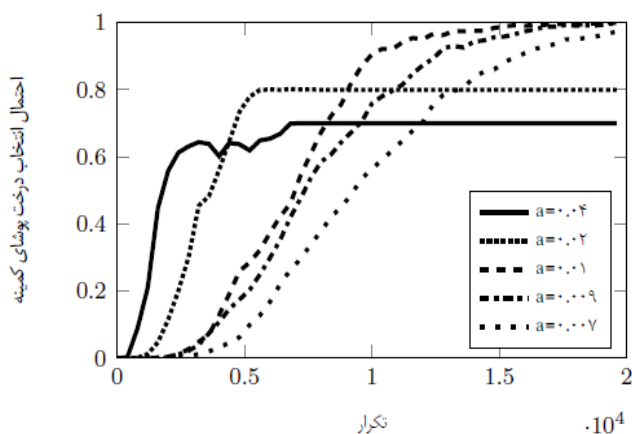
شکل ۹: نحوه تغییر احتمال انتخاب درخت پوشای کمینه در الگوریتم [۱۶] به ازای مقادیر مختلف نرخ یادگیری.
