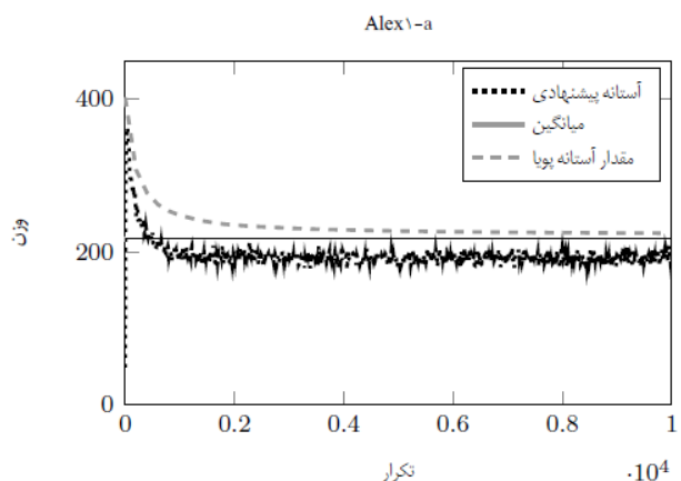
شکل ۵: مقایسه مقادیر مورد استفاده در ارزیابی اقدامات یادگیری آتاماتا در الگوریتم ارائه شده در [۱۶] و الگوریتم ۱ پیشنهادی در مقایسه با میانگین وزن درخت پوشای بهینه (نرخ یادگیری ۰/۰۰۷ بوده است).
