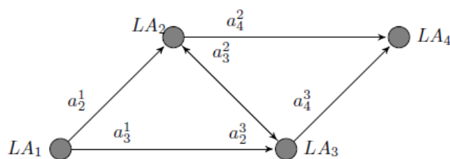
شکل ۲: آتاماتای یادگیر توزیع‌شده.
